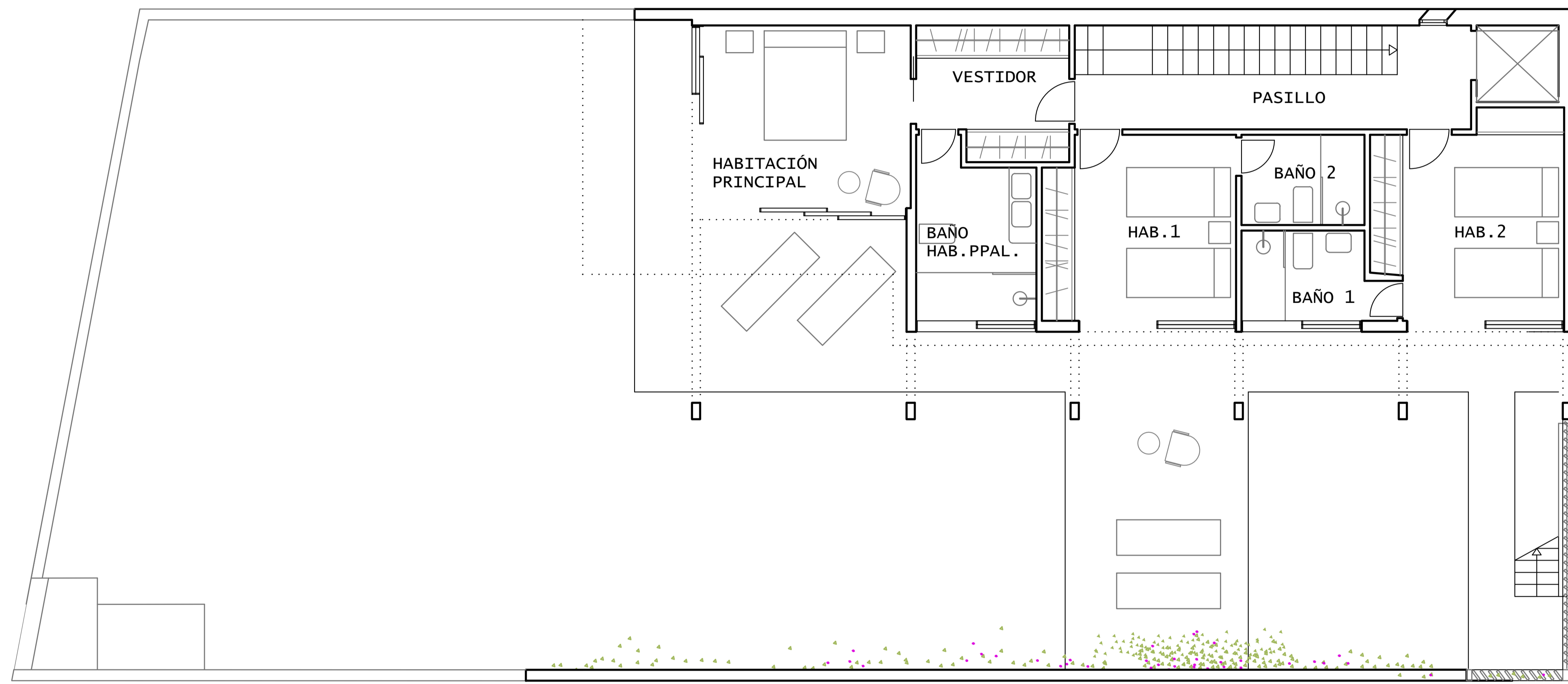
PLANTA PRIMERA E:1/150
