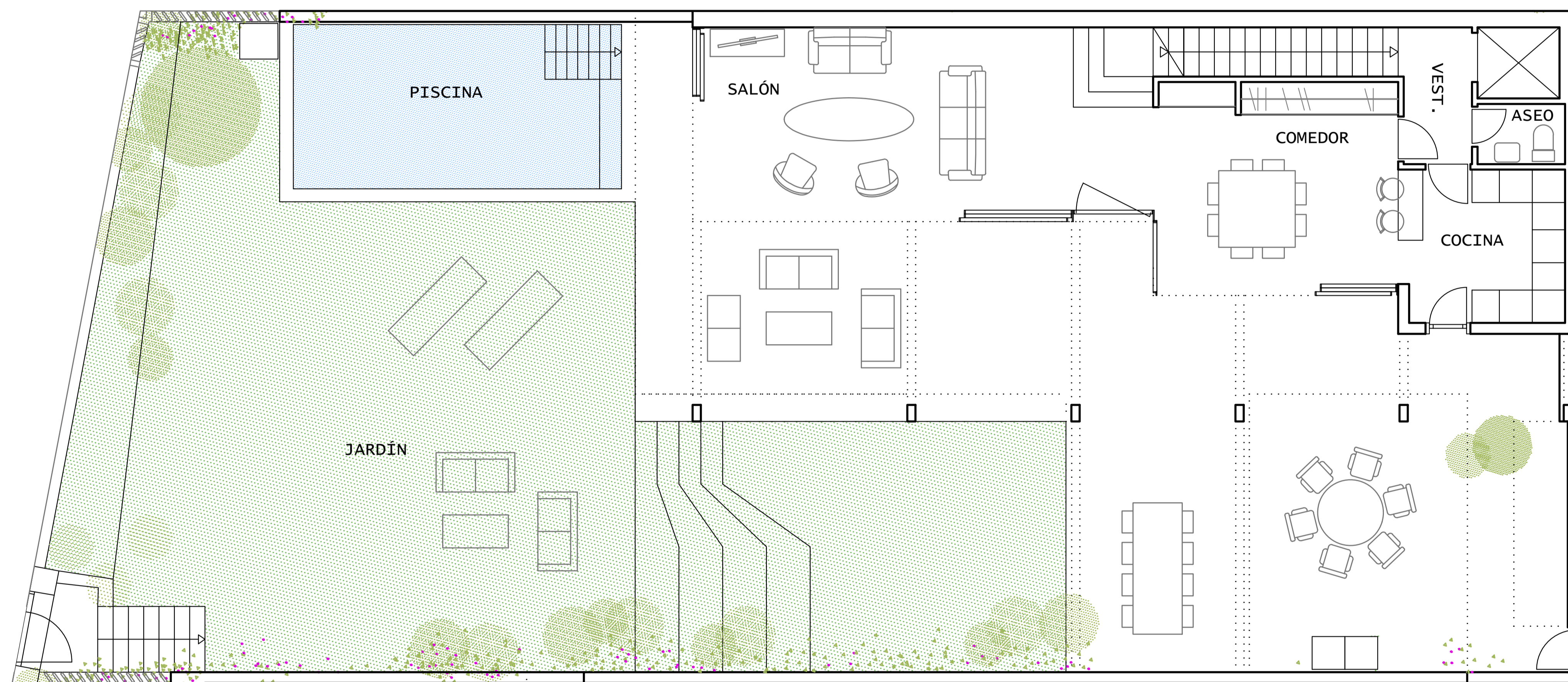
PLANTA BAJA E:1/150
