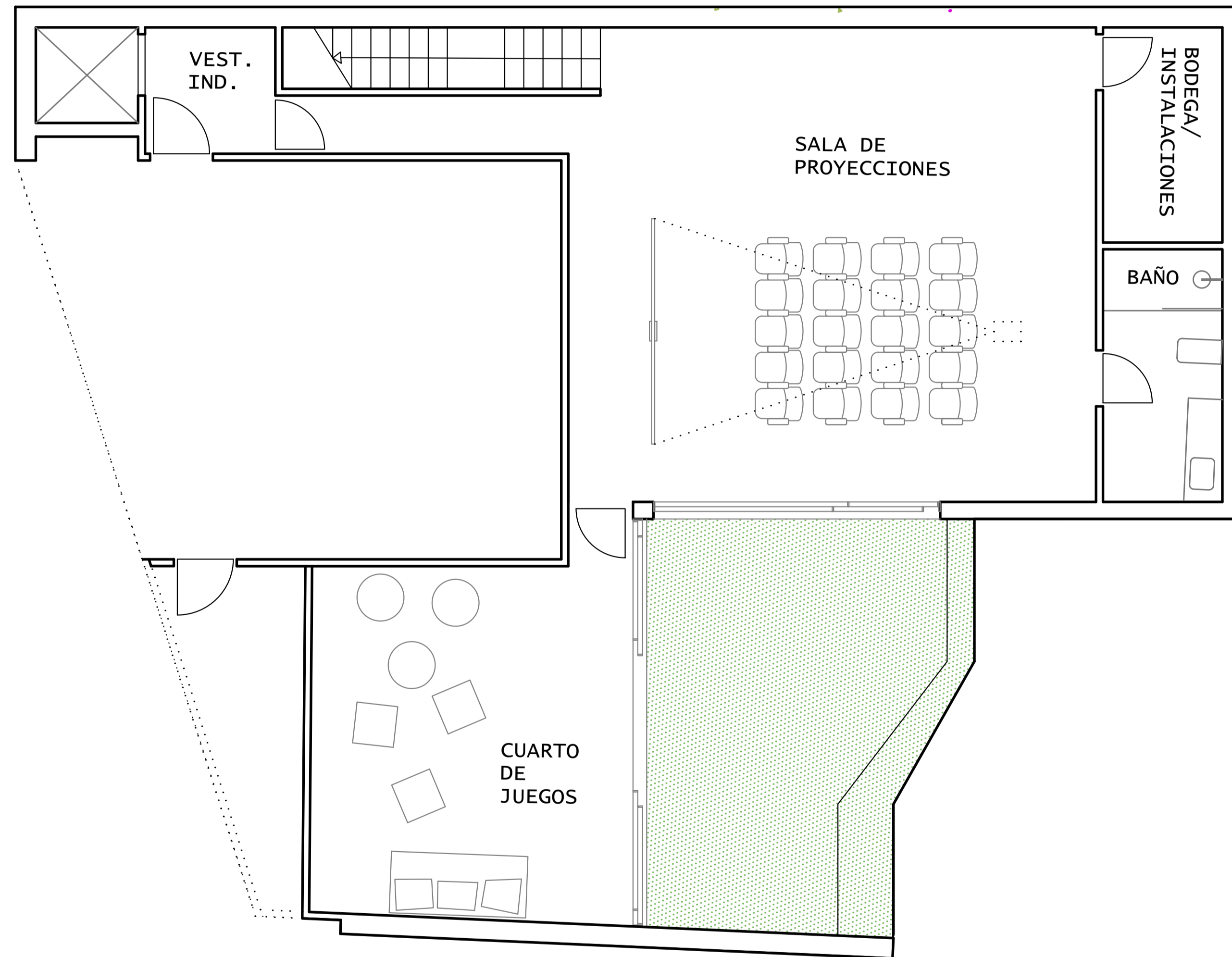
PLANTA PATIO E:1/150
